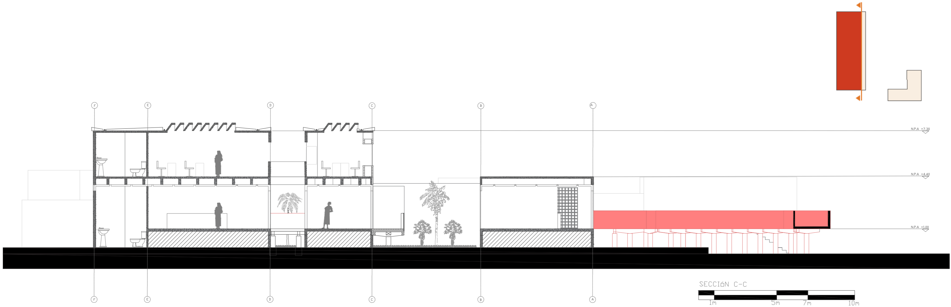
Figura 28: Sección C-C. (fuente: Elaboración propia)
