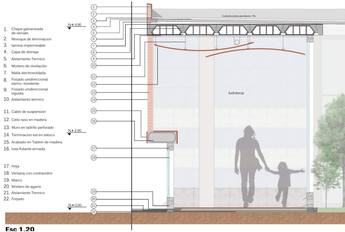
Figura 135. Detalle constructivo fachada norte .
