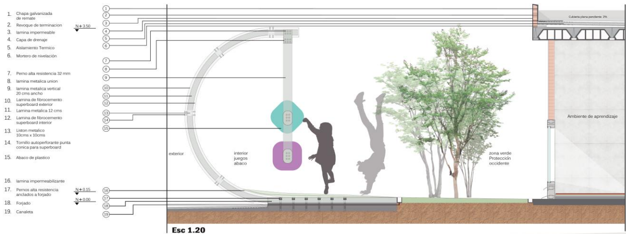
Figura 136. Detalle constructivo muro cerramiento.
