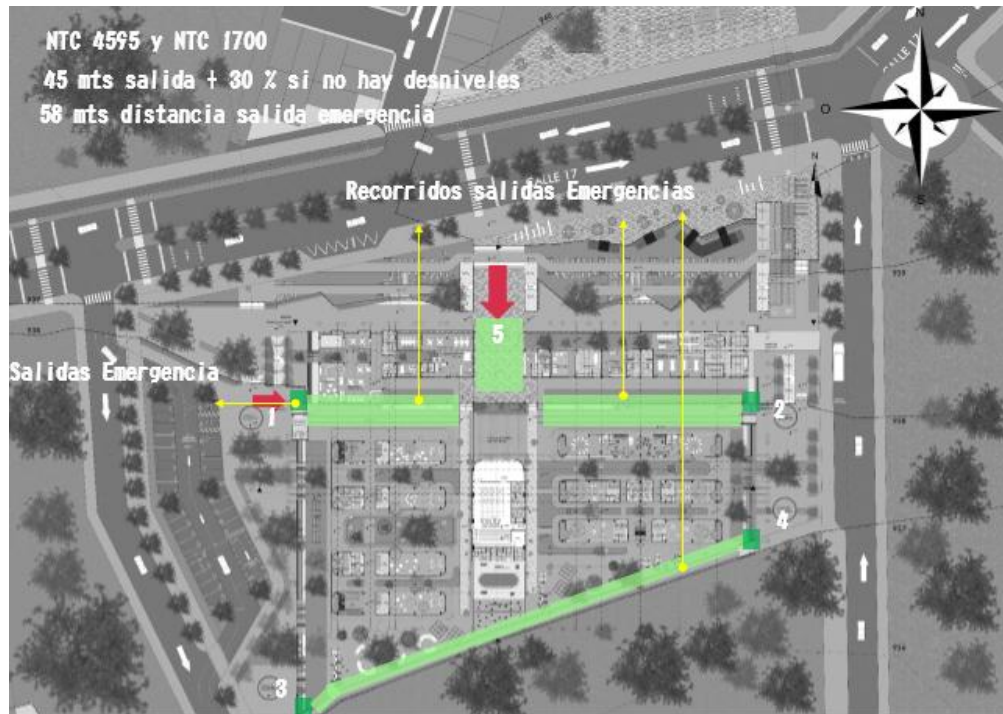
Figura 83. Esquema de salidas de emergencia del proyecto
