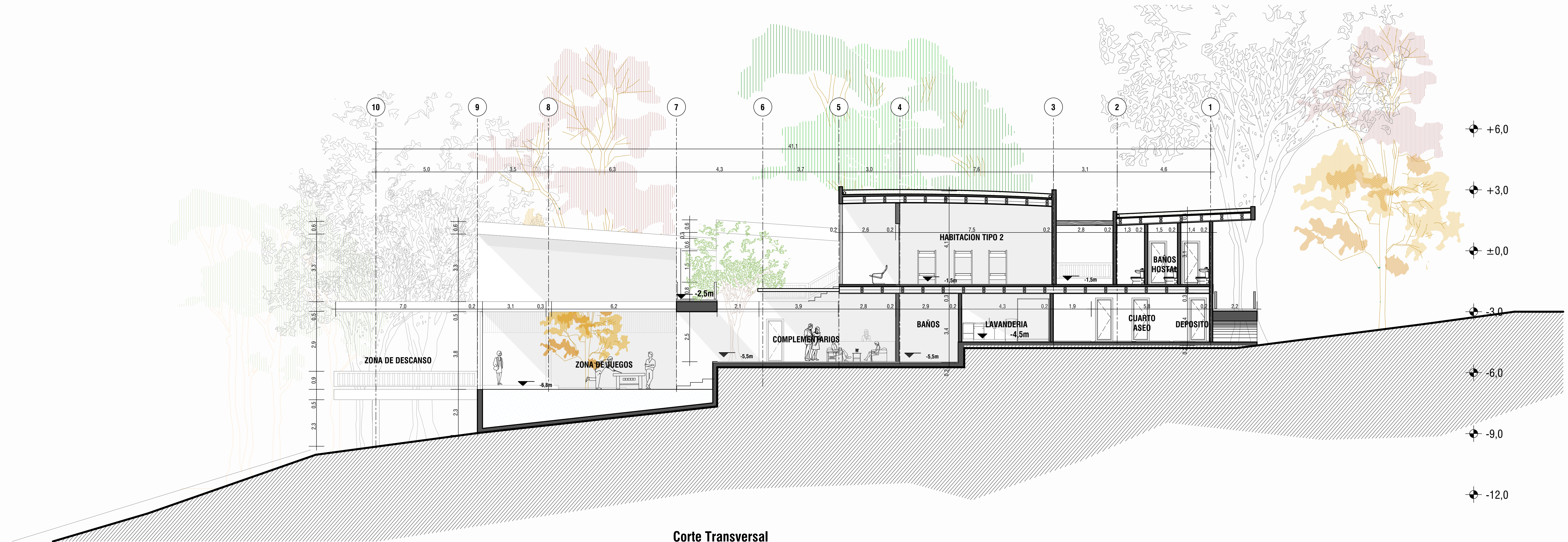
Corte Transversal Sección C-C Esc 1:100
