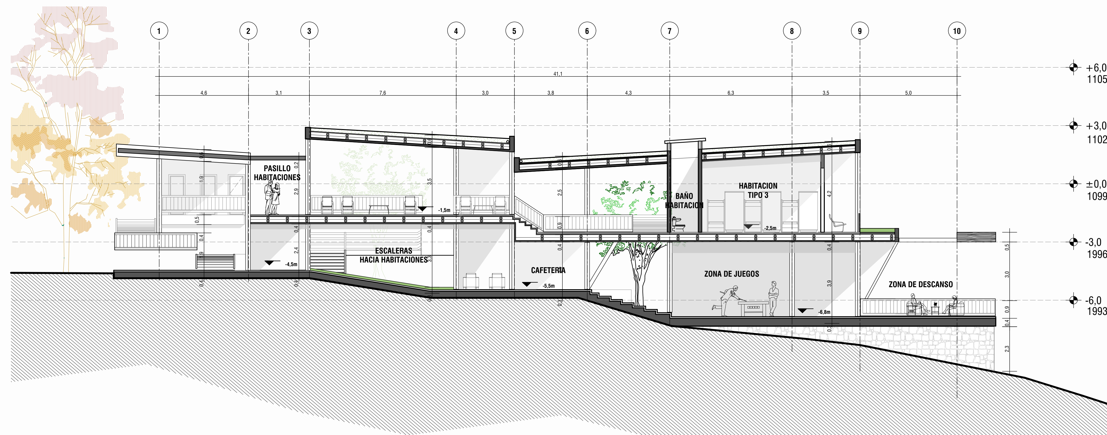
Corte Transversal Sección D-D Esc 1:100
