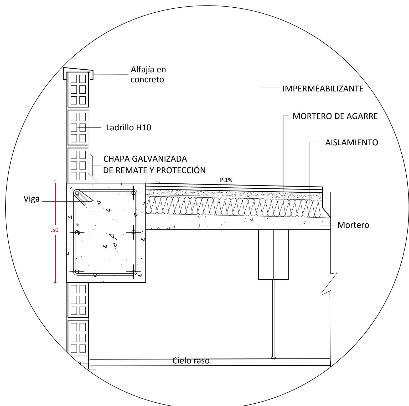
Cubierta ligera con losa
