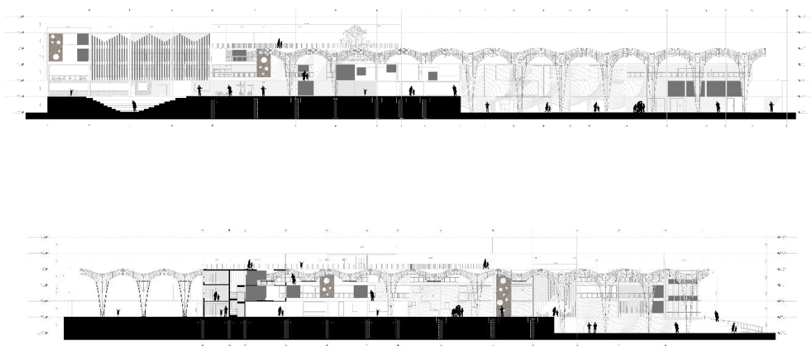
Ilustración 26. Fachadas arquitectónicas
