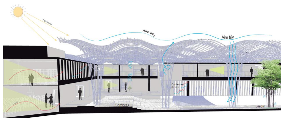
Ilustración 20. Estrategias bioclimáticas
