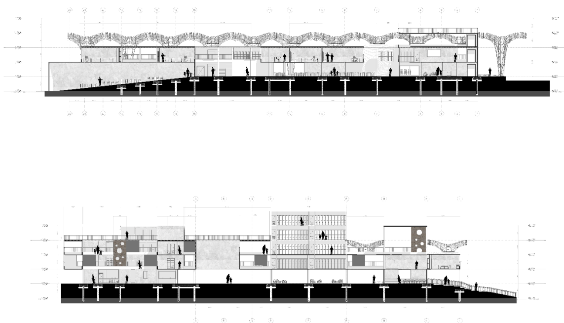
Ilustración 25. Cortes arquitectónicos
