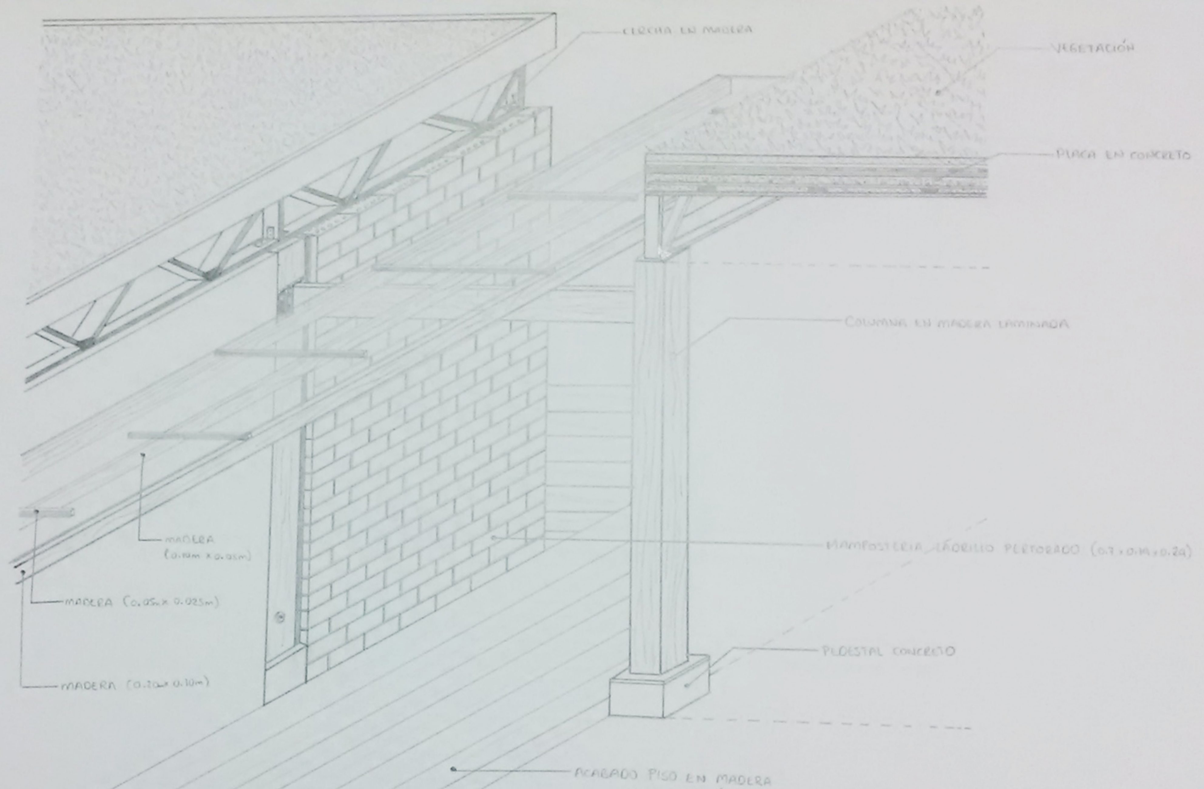
DETALLE PERSPECTIVA PERGOLA ESC. 1:20
