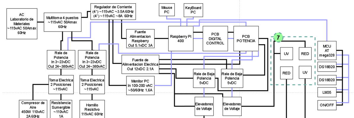
Figura 52. Diagrama de bloques sección 7.
