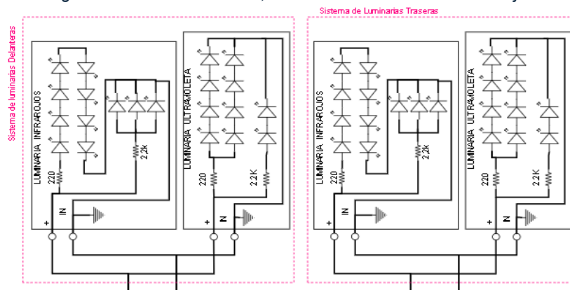
Figura 57. Circuito sección 7, Luminarias Ultravioleta e Infrarroja.
