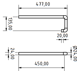
Figura 9. Boquillas para la Salida del Vapor.
