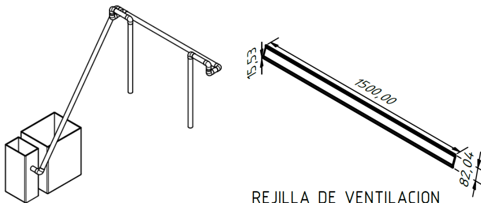
Figura 8. Sistema para Vaporizar el agua y rejilla de ventilación
