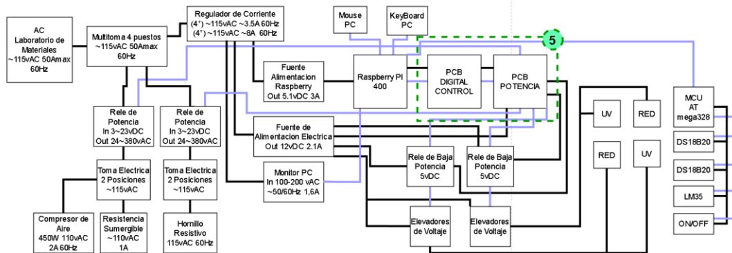
Figura 45. Diagrama de bloques sección 5.
