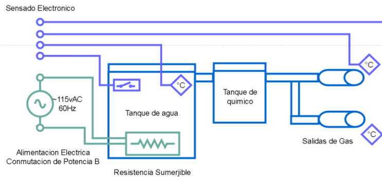
Figura 35. Circuito de tubería de vapor de agua y generación de la niebla salina.
