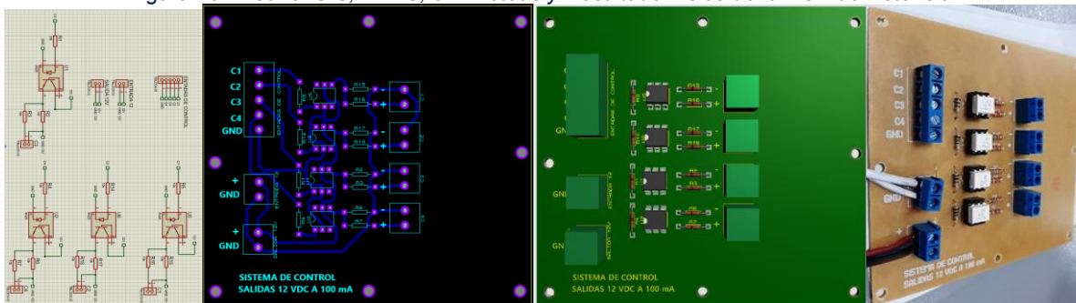
Figura 49. Diseño ISIS, ARES, 3D Proteus y Resultado Físico de la PCB de Potencia.
