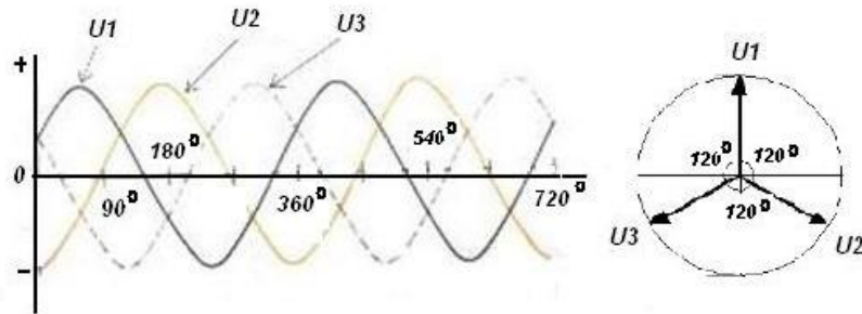
Figura 23. Representación de Corriente alterna Trifásica.
