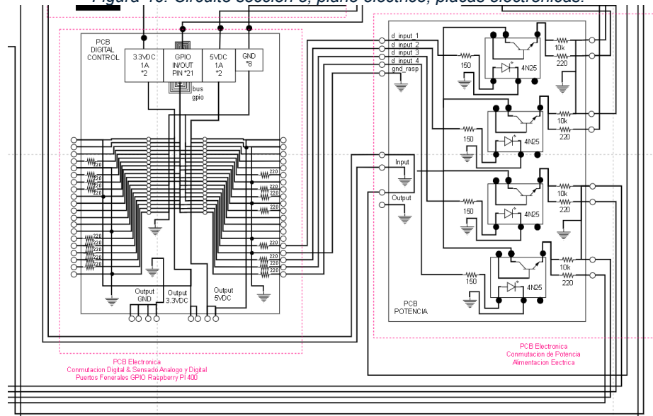
Figura 46. Circuito sección 5, plano eléctrico, placas electrónicas.
