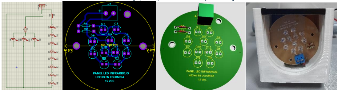
Figura 53. Diseño de Luminaria con luz Infrarroja, ISIS, ARES 3D en proteus y resultado en físico con carcaza en 3D.
