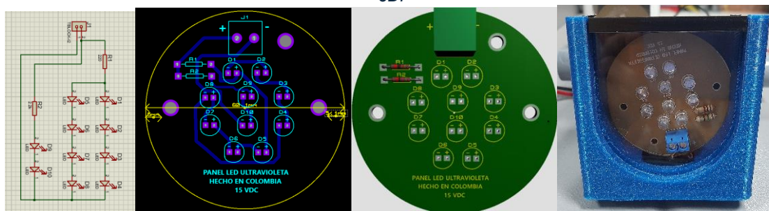
Figura 54. Diseño de circuito de luz ultravioleta, ISI, ARES, 3D Proteus y Resultado Físico con Protección impresa en 3D.
