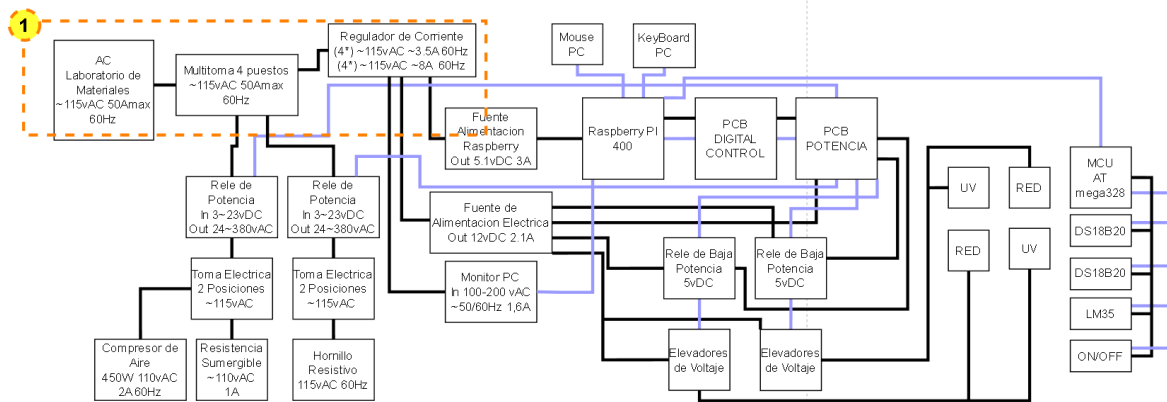
Figura 27. Diagrama de bloques sección 1.
