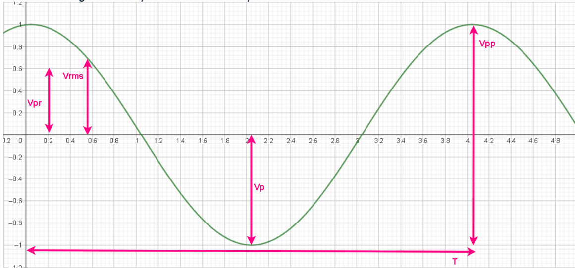
Figura 18. Representación de las partes de una onda Senoidal de una red Eléctrica.
