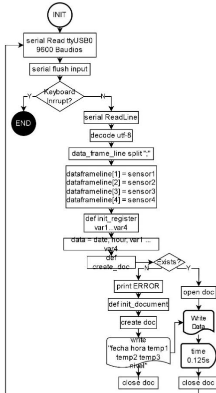
Anexo 4. Diagrama de software, Lectura Sensores MCU ATmega32 Arduino Nano.
