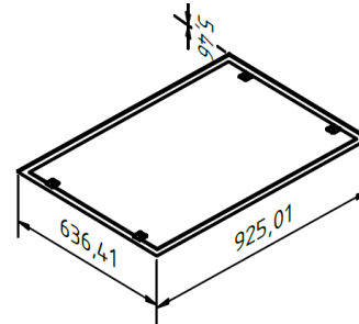
Figura 5. Cuba en Vidrio Refractario y Vidrio Polarizado.
