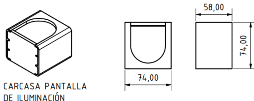
Figura 11. Carcasa impresa en 3D, Pantalla de Iluminación Ultravioleta e Infrarroja.
