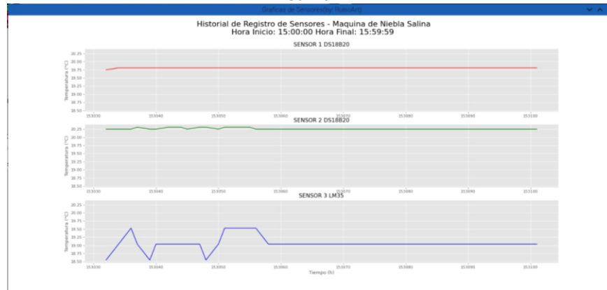
Figura 70. Interfaz de Registros, Gratificación de sensores de temperatura implementados en la Máquina de Niebla Salina.
