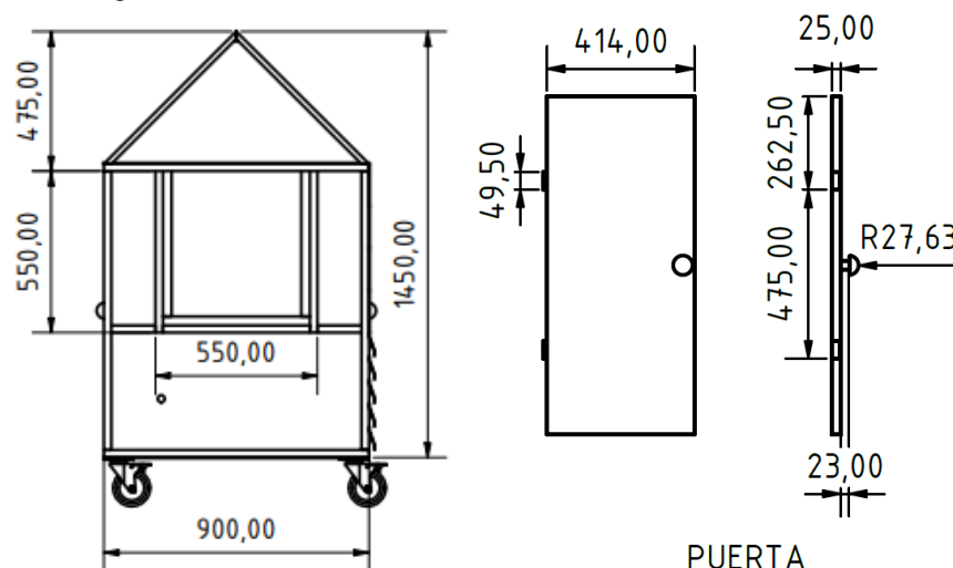
Figura 4. Plano General de la Cámara de Niebla Salina vista frontal.
