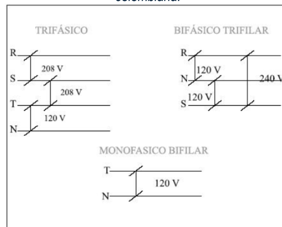
Figura 22. Clasificación de hilos de alimentación según su tipo en red de Lower Voltage. Redes de distribución colombiana.
