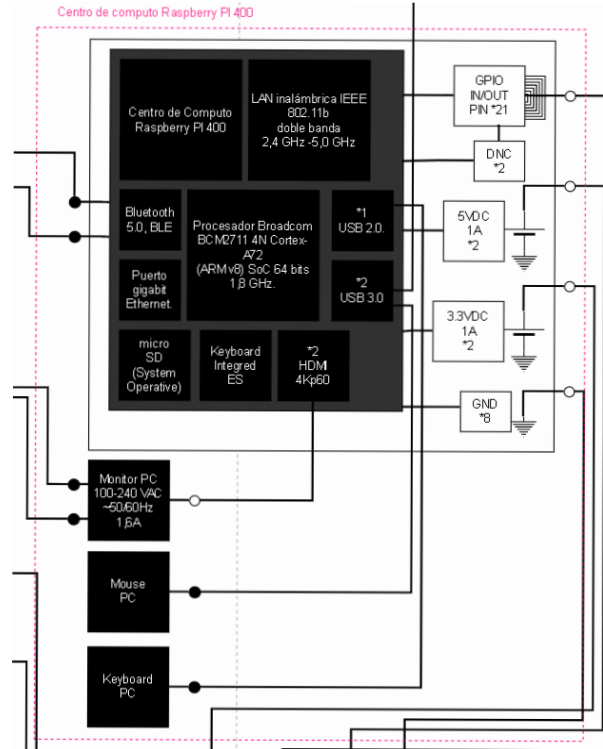
Figura 44. Circuito sección 4, Centro de Computo Raspberry PI 400.
