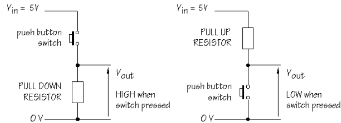
Figura 64. Configuración para switch PULL-UP y PULL-DOWN.
