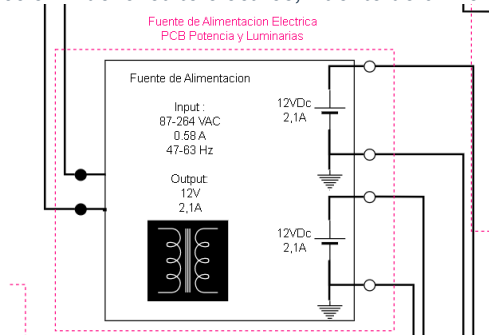
Figura 41. sección 4 del circuito eléctrico, Fuente de alimentación AC/DC.
