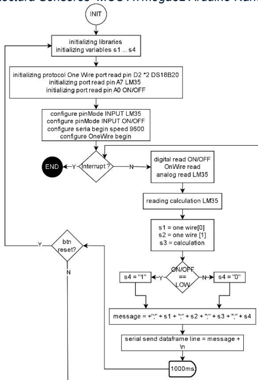
Anexo 4. Diagrama de software, Lectura Sensores MCU ATmega32 Arduino Nano.
