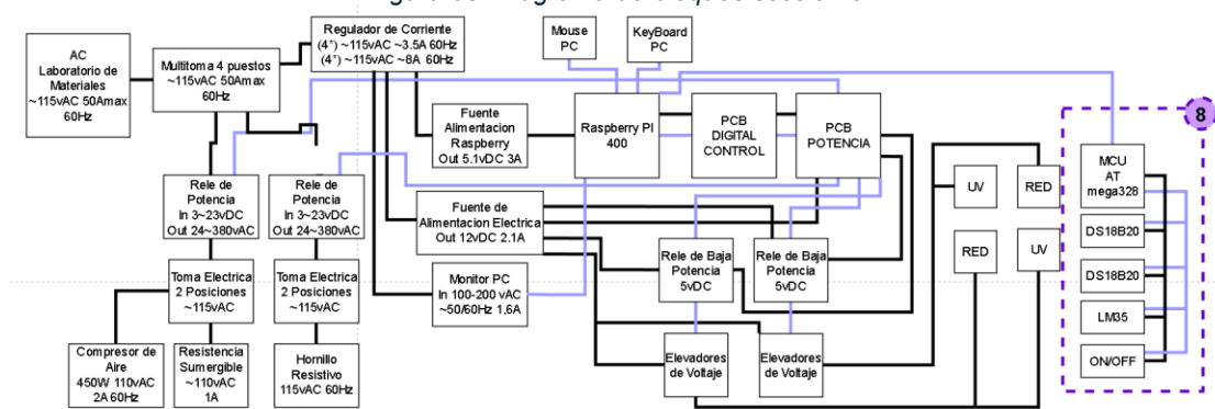
Figura 58. Diagrama de bloques sección 8.
