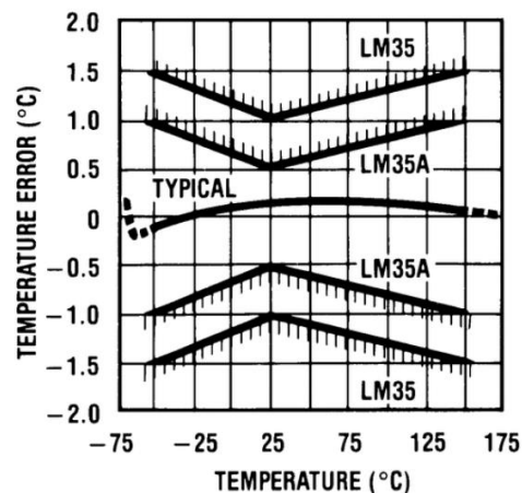
Figura 63. Error de medición en rango de trabajo de temperatura para sensor LM35.
