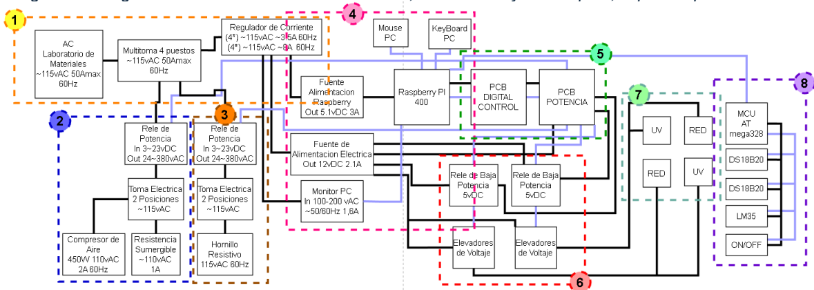
Figura 26. Diagrama General de conexiones eléctrica, electrónicas y de cómputo, separado por secciones.
