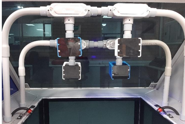
Figura 56. Brazos de suspensión de luminarias traseras y delanteras.
