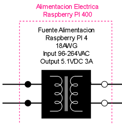
Figura 40. sección 4 del plano eléctrico, alimentación eléctrica de la Raspberry PI 400.
