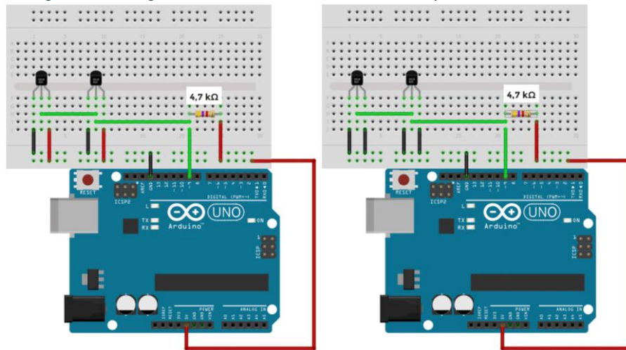
Figura 62. configuración de conexión de alimentación para sensor DS18B20.
