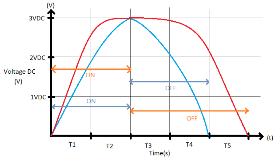
Figura 73. Diagrama realizado a mano para representar el arreglo en retardos con la implementación de librerías diferentes para la comunicación con la GPIO de la Raspberry PI.
