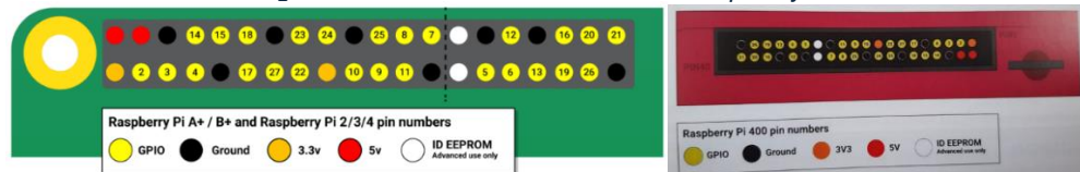
Figura 42. Puerto estándar GPIO de Raspberry PI.
