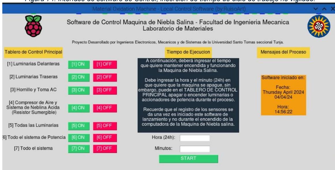
Figura 74. Interface de software de Control, inserción de tiempo de ciclo de trabajo no vigilado.
