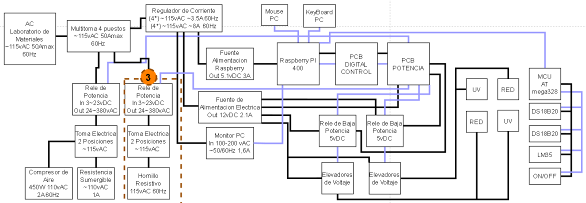
Figura 37. Diagrama de bloques sección 3.
