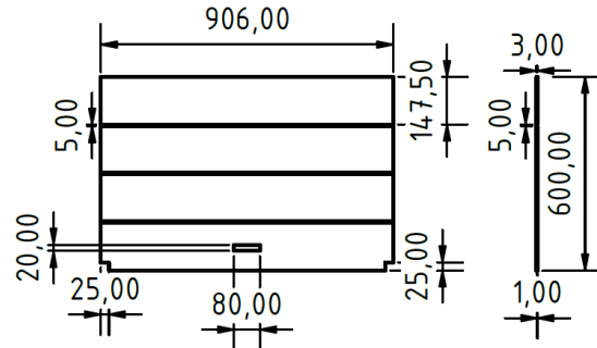
Figura 3. Tapa Superior para el Equipo de cómputo.
