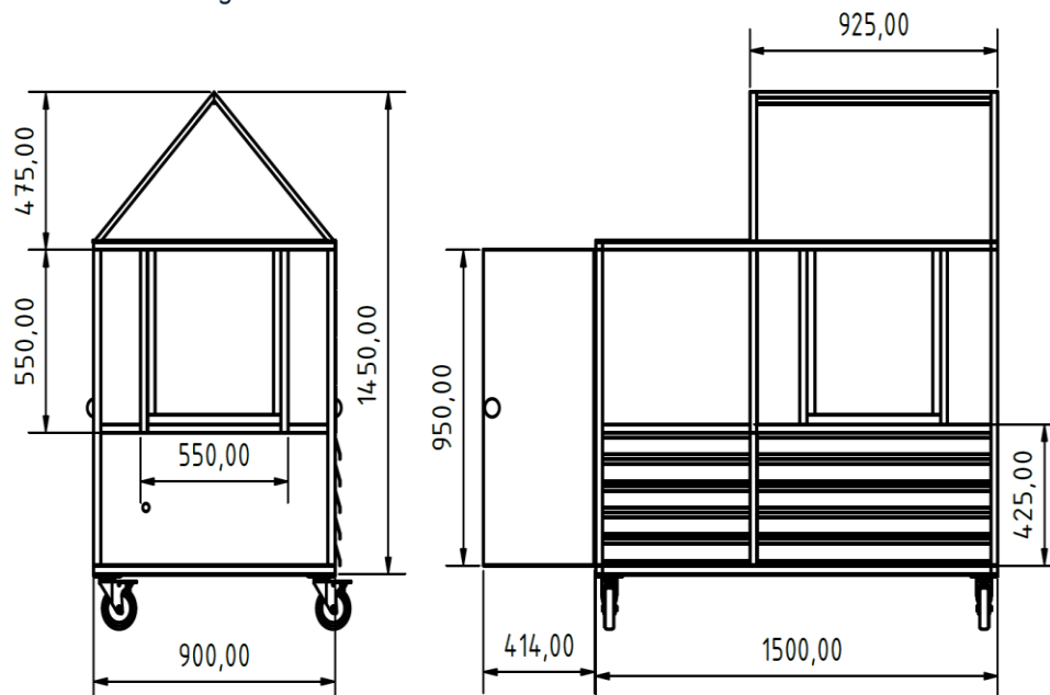
Figura 12. Plano General de la Cámara de Niebla Salina.
