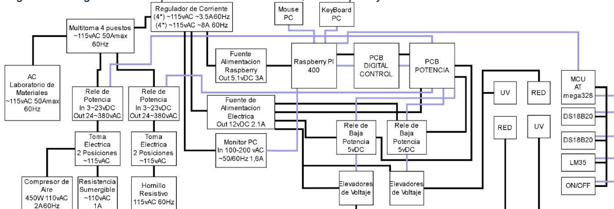
Figura 17. Diagrama de Bloques del Sistema Eléctrico, de cómputo y electrónico de la Cámara de Niebla Salina.
