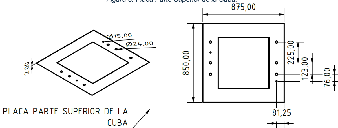
Figura 6. Placa Parte Superior de la Cuba.
