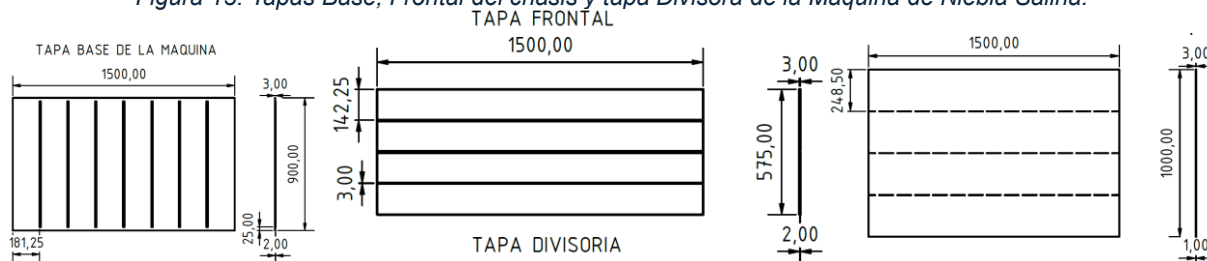
Figura 13. Tapas Base, Frontal del chasis y tapa Divisora de la Máquina de Niebla Salina.
