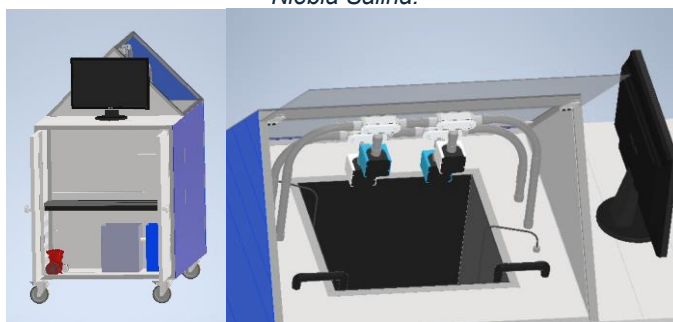
Figura 15. Representación frontal en visualización 3D del prototipo y Representación Parte Superior Cámara de Niebla Salina.
