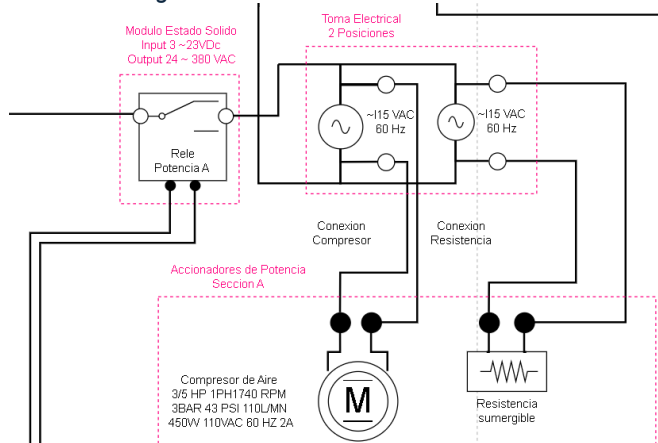
Figura 34. Circuito eléctrico sección 2.
