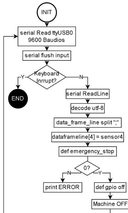
Anexo 2. Diagrama de Software, Botón de emergencia.
