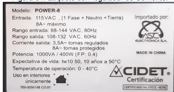
Figura 31. Etiqueta del Regulador de Corriente.
