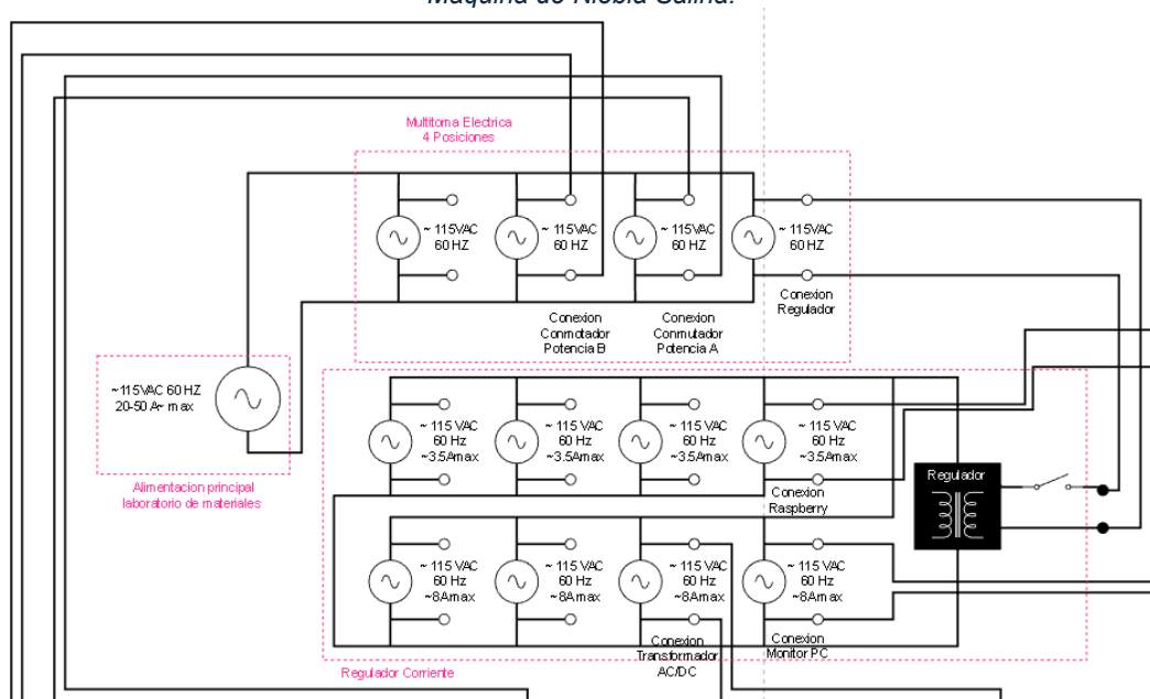
Figura 32. Circuito sección 1 del Diagrama Completo de conexiones eléctricas, electrónicas y de cómputo de la Máquina de Niebla Salina.
