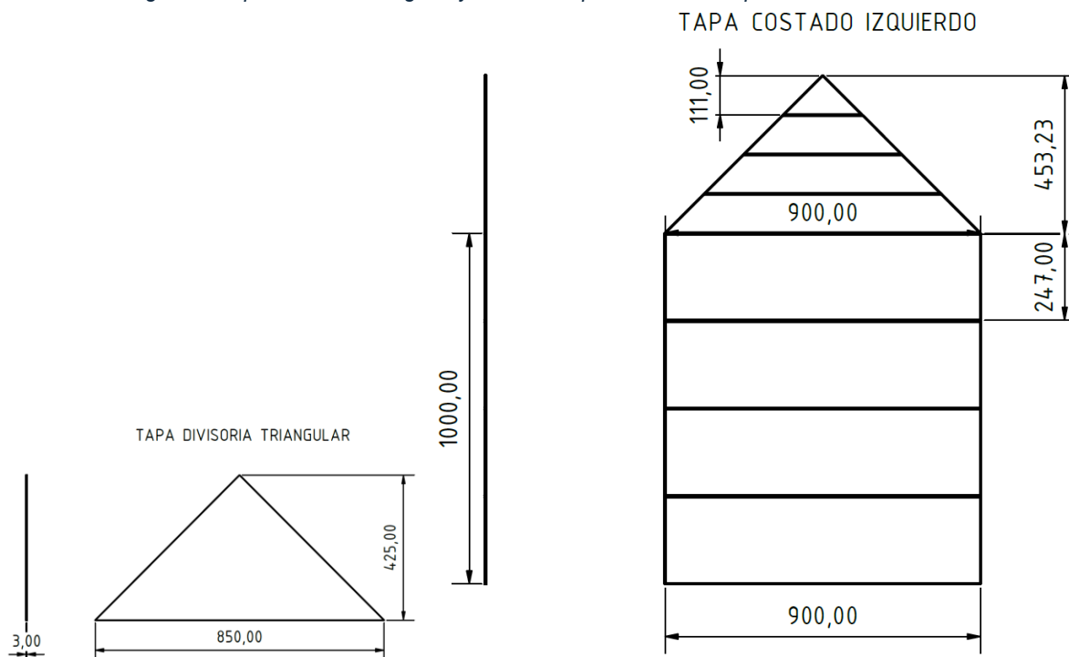
Figura 7. Tapa divisora Triangular y costado izquierdo de la Máquina de Niebla Salina.
