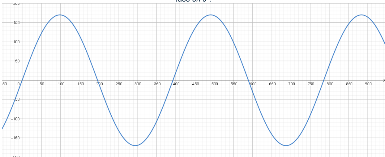
Figura 19. Representación en GeoGebra de red monofásica representa una red de 120VrmsAC, 60Hz o 0,016s con fase en 0^\circ .
