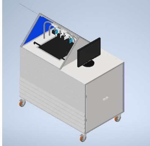
Figura 16. Representación Lateral de la Cámara de Niebla Salina.
