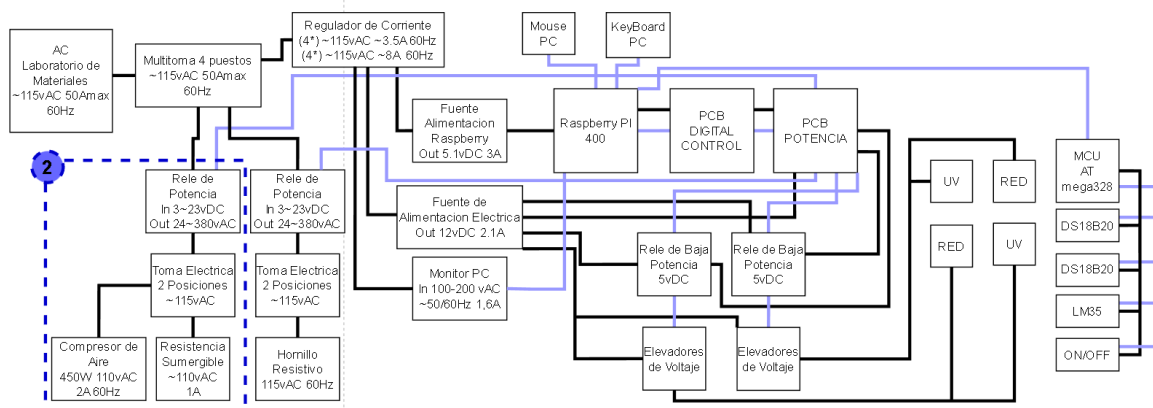
Figura 33. Diagrama de bloques sección 2.
