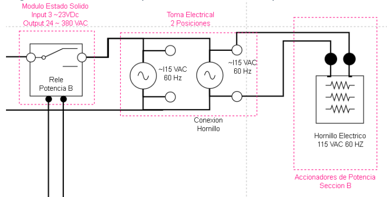
Figura 38. Sección 3 del plano eléctrico de la Máquina de Niebla Salina.
