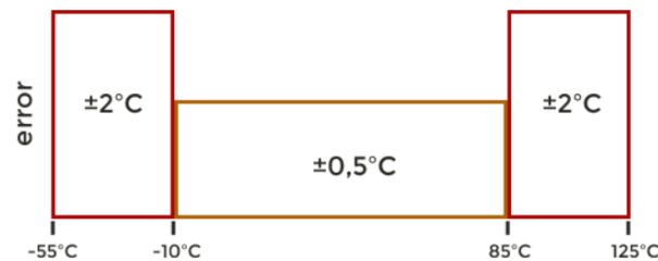
Figura 60. Error de medición por rango de Trabajo en Temperatura, sensor DS18B20.
