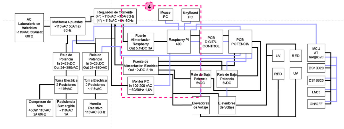
Figura 39. Diagrama de bloques sección 4.
