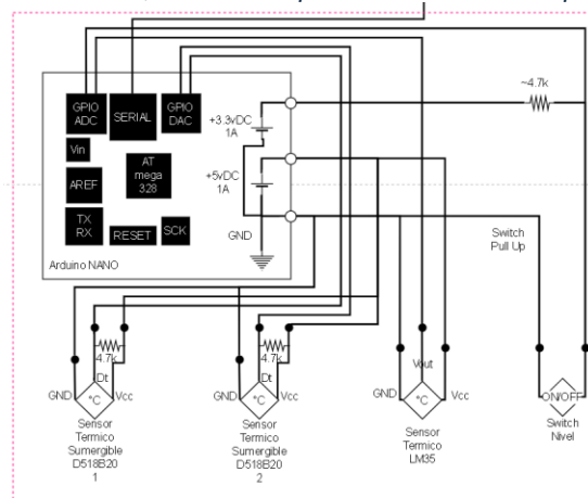
Figura 59. Circuito sección 8, sensores implementados en la Máquina de niebla salina.
