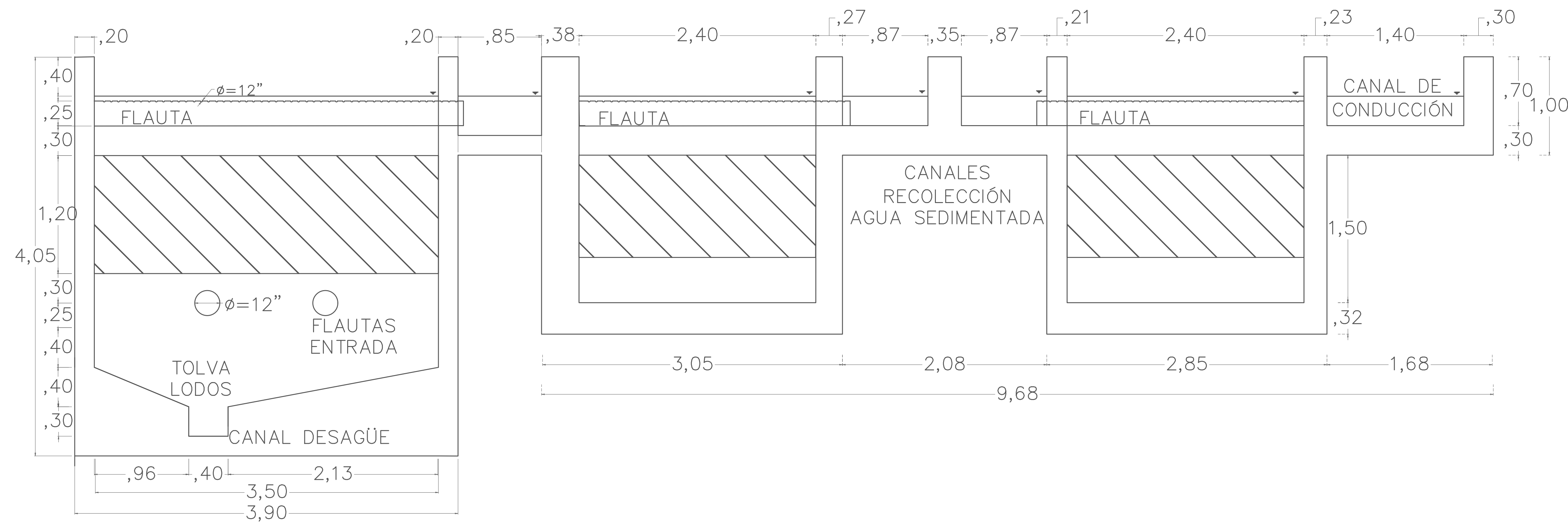
PERFIL TRANSVERSAL SEDIMENTACIÓN CORTE F—F
