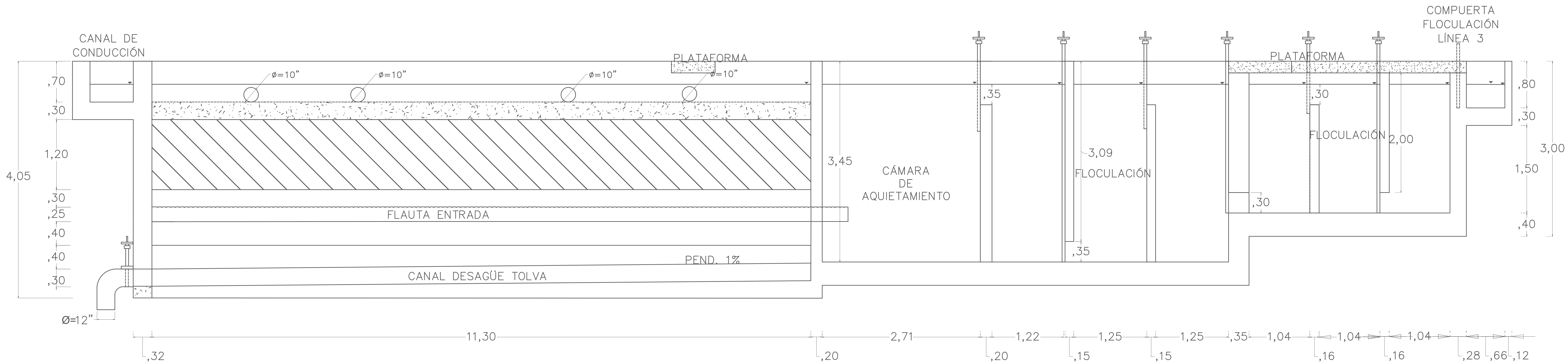
PERFIL LONGITUDINAL FLOCULACION Y SEDIMENTACIÓN CORTE E—E
