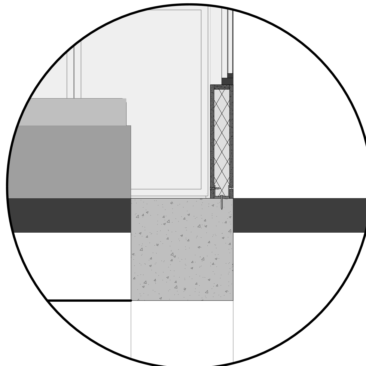
DETALLE MURO PLYCEM
