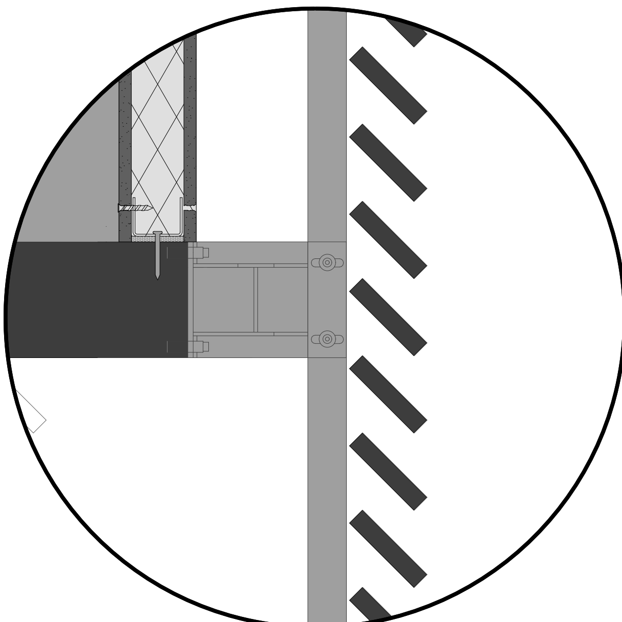
DETALLE DOBLE PIEL
