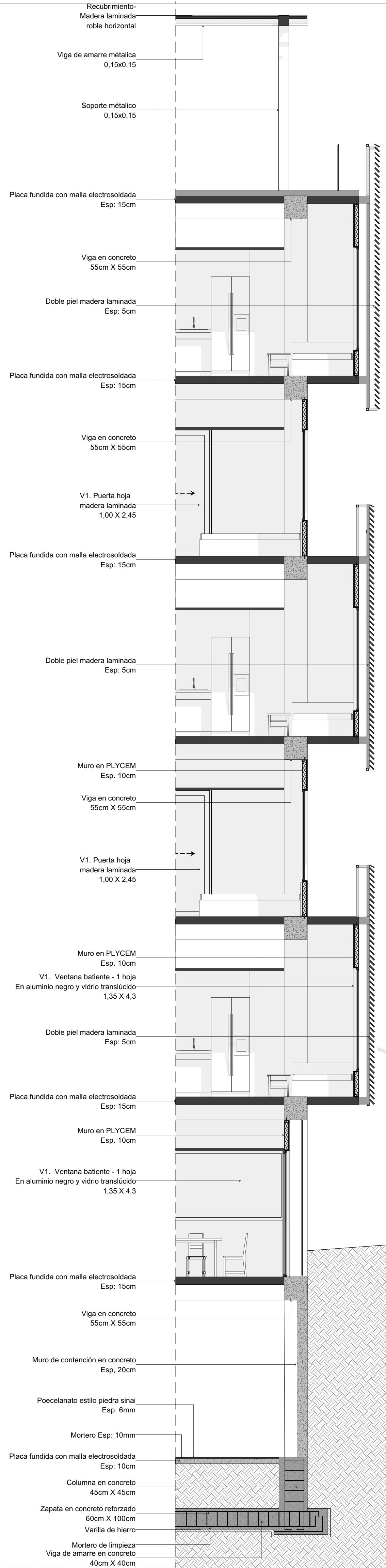
CORTE FACHADA B'B
