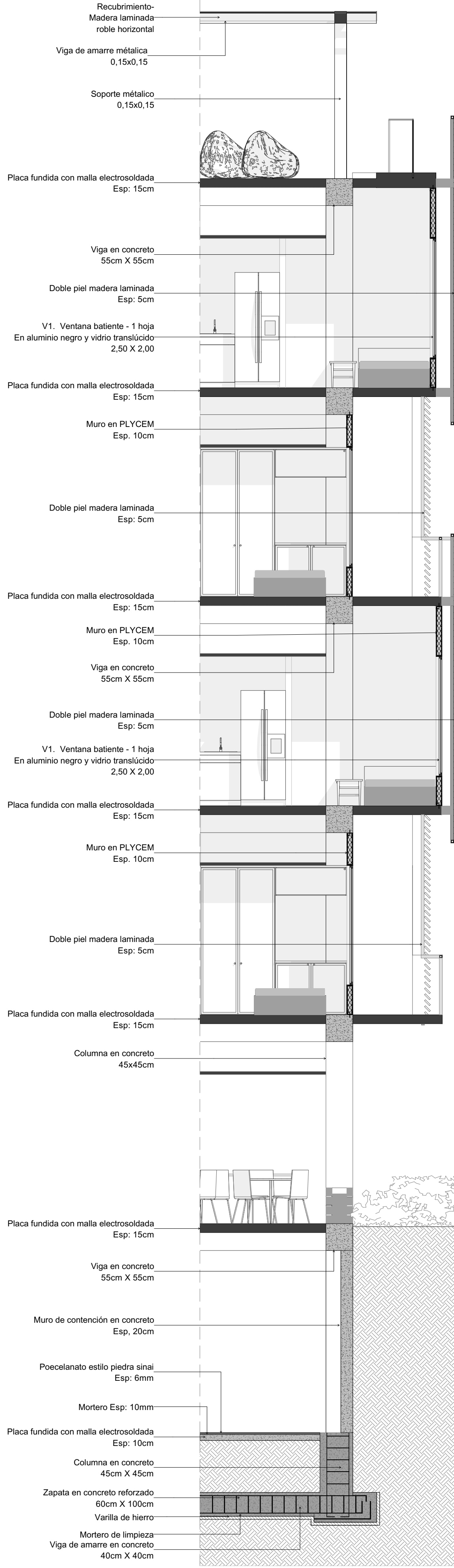
CORTE FACHADA A'A
