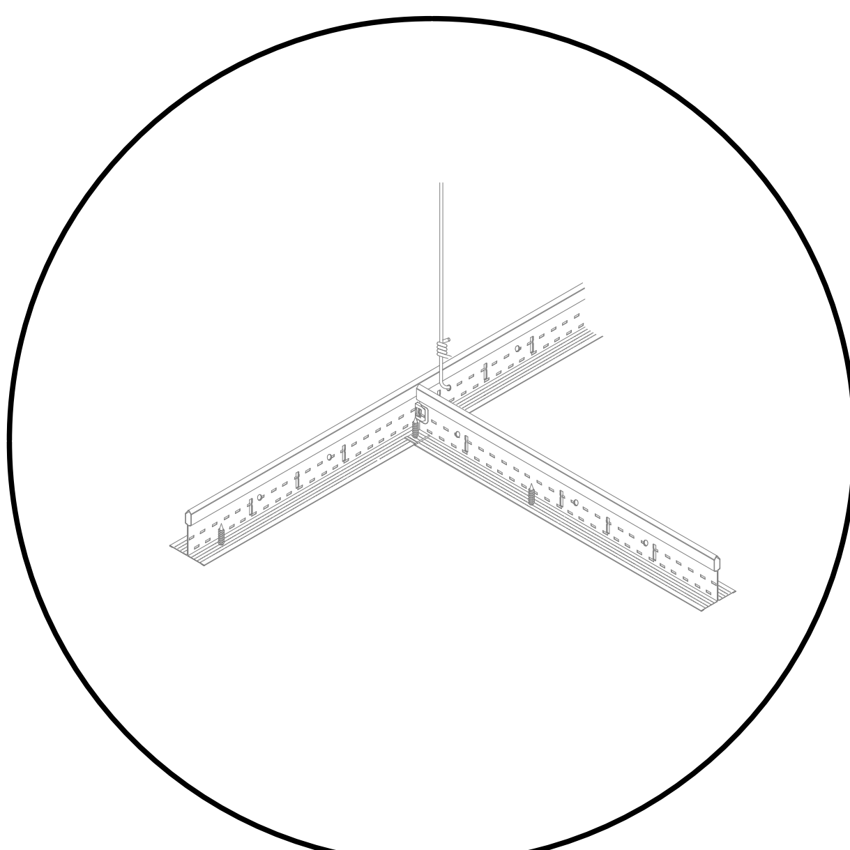
DETALLE CIELO RASO GYPSUM
