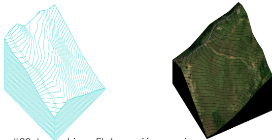
Figura #28 Isometrico- Elaboración propia
