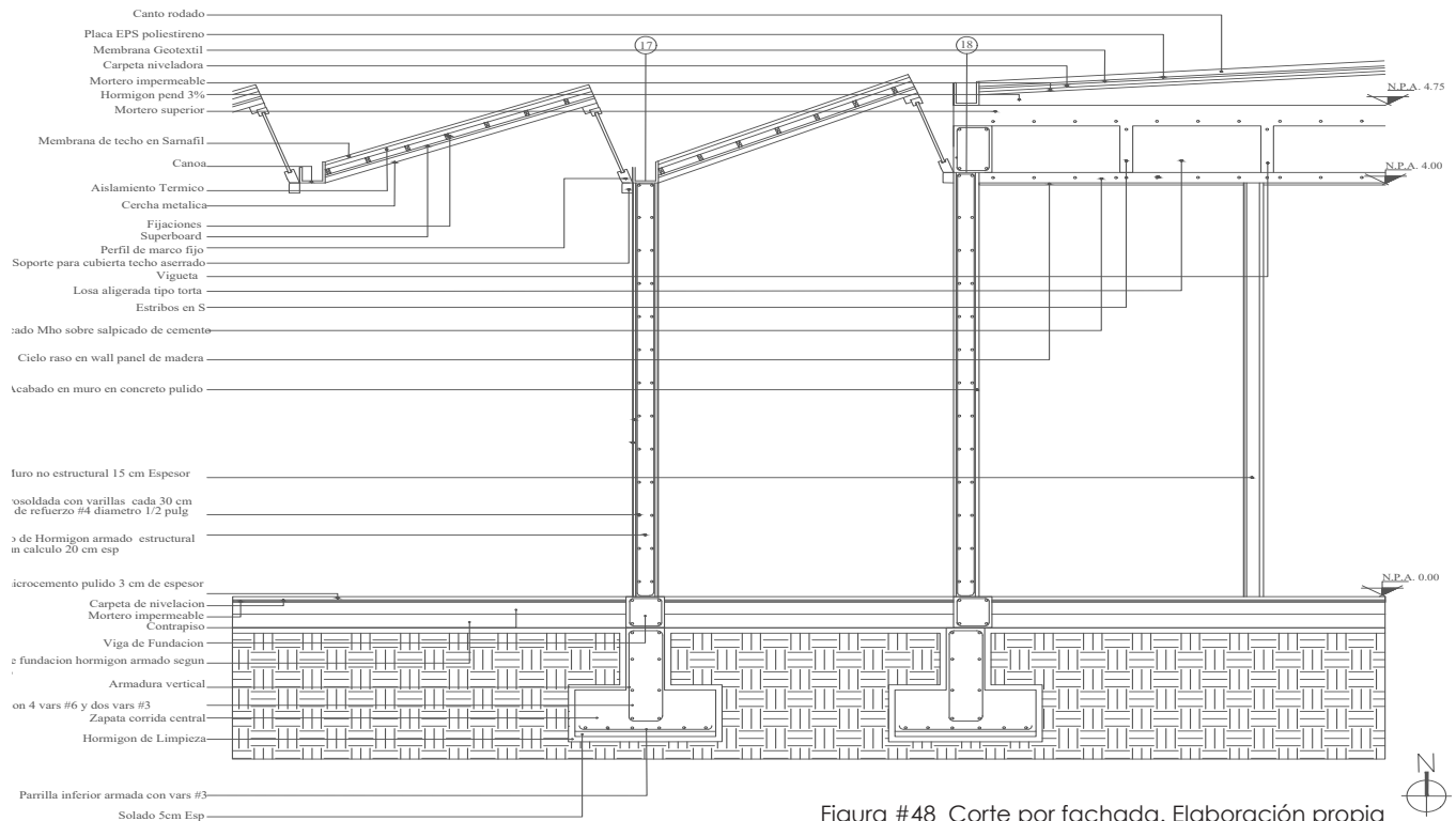
Figura #48 Corte por fachada. Elaboración propia
