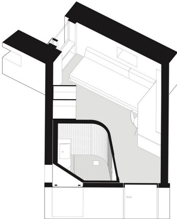
Figura #14 Prisión Storstrom ArchDaily 2017- Isométrico celda
