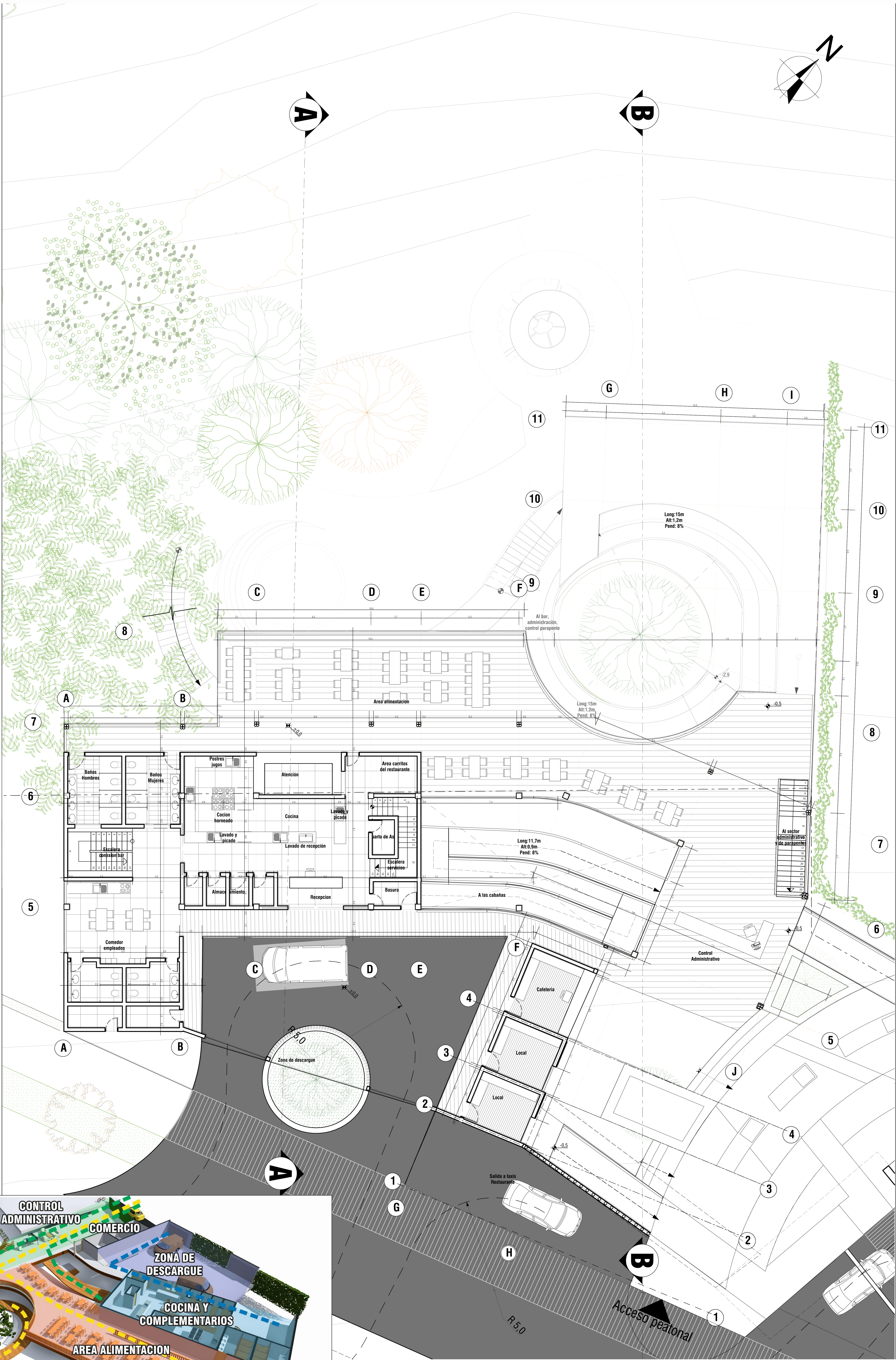
Planta Acceso Bloque A Esc_1:100
