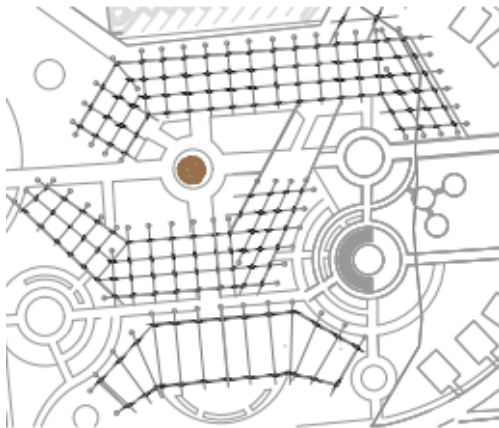
Imagen 45. Planta estructural. Fuente: Autores
