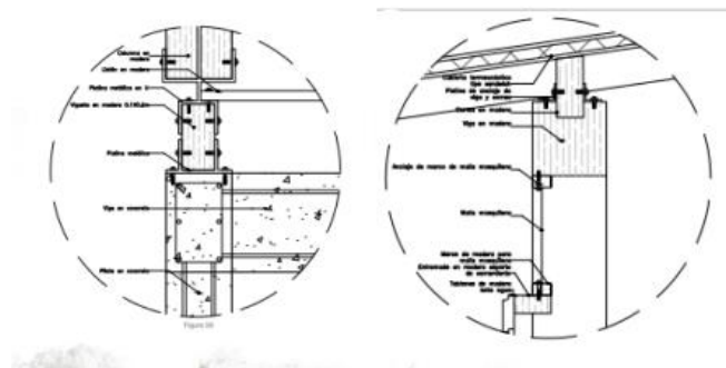
Imagen 46. Detalle constructivo. Fuente: (Facultad De Arquitectura et al., n.d.)
