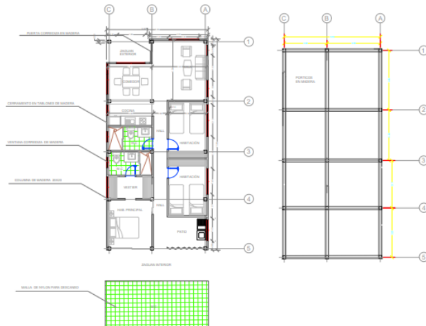
Imagen 48. Planta vivienda palafítica. Fuente: Autores
