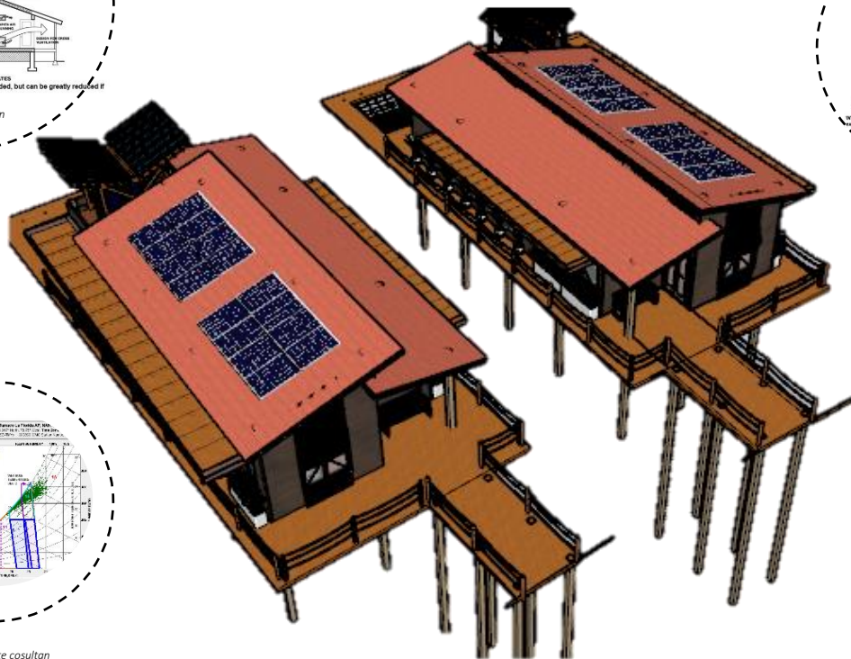
Imagen 50. Perspectiva vivienda palafítica. Fuente: Autores
