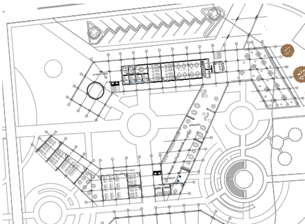
Imagen 42. Planta segundo piso. Fuente: Autores
