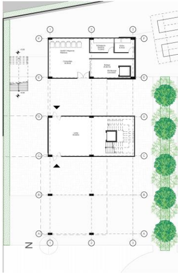
PRIMER PISO
